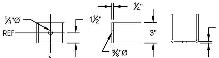
DETAIL F1 OPGW DOWNLEAD TAB
