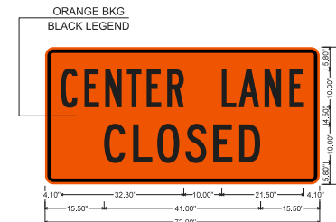
WZ-W20-5R SIGN
