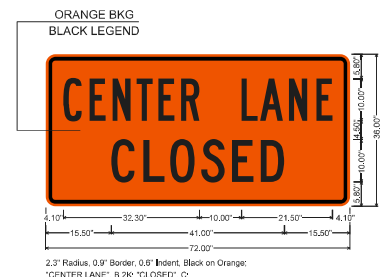
WZ-W20-5C SIGN
