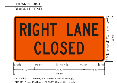
WZ-W20-5R SIGN
