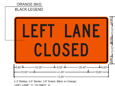
WZ-W20-5L SIGN
