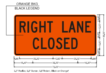
WZ-W20-5R SIGN
