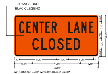
WZ-W20-5C SIGN
