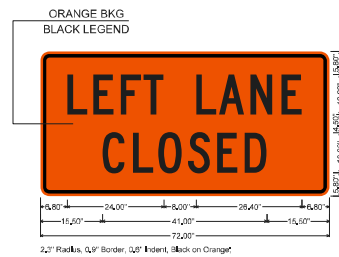
WZ-W20-5L SIGN
