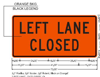
WZ-W20-5L SIGN
