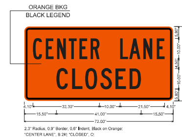
WZ-W20-5C SIGN
