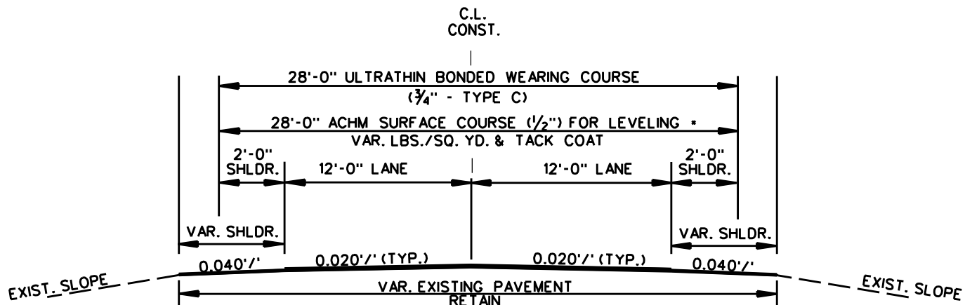
2 LANE OPEN SHOULDER U.T.B.W.C. OVERLAY (4'-0" SHLDR.)
