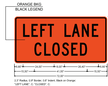
WZ-W20-5L SIGN
