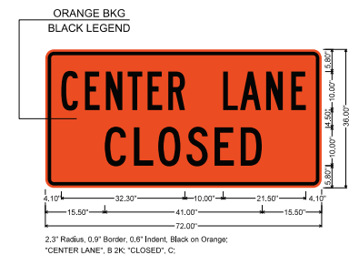
WZ-W20-5C SIGN
