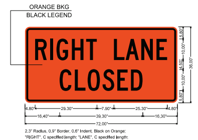
WZ-W20-5R SIGN
