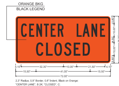
WZ-W20-5C SIGN
