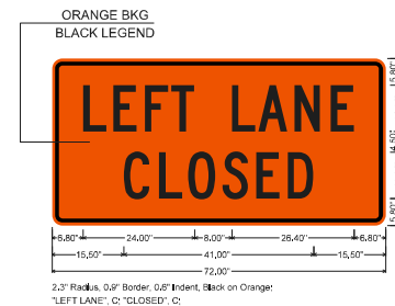
WZ-W20-5L SIGN
