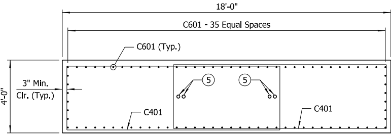
SECTION B-B Scale: 3/8" = 1'-0"
