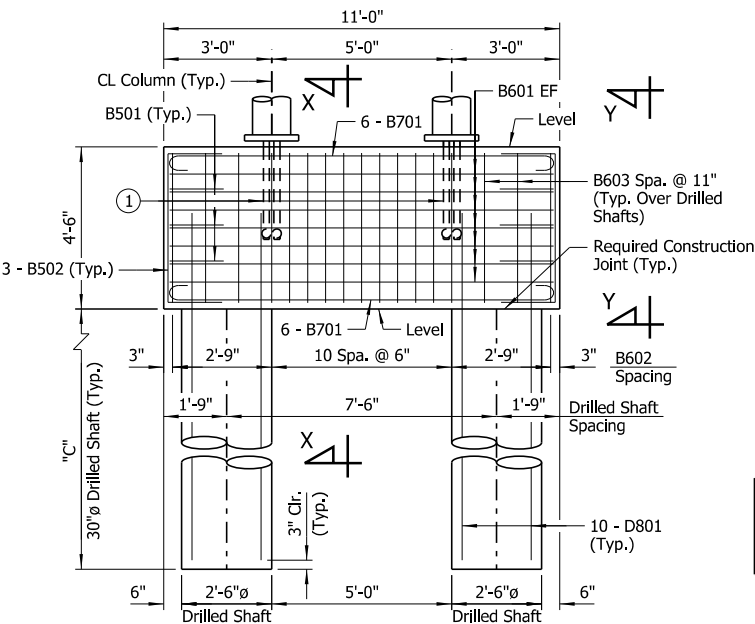
VIEW V-V Scale: ¾" = 1'-0"
