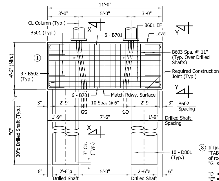
VIEW W-W Scale: ¾" = 1'-0"
