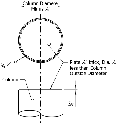
END CAP DETAIL Scale: 1 1/2" = 1'-0"
