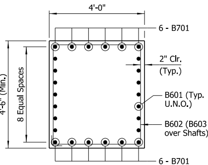
SECTION X-X Scale: ½" = 1'-0"
