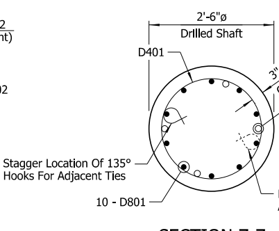
SECTION Z-Z Scale: ¾" = 1'-0"
