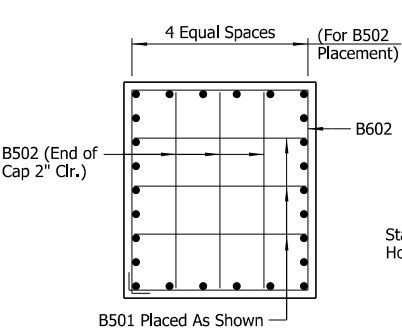
VIEW Y-Y Scale: ½" = 1'-0"
