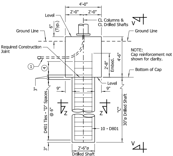
ELEVATION - FOUNDATION A2 ② Scale: ¾" = 1'-0"
