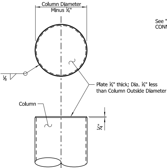
END CAP DETAIL Scale: 1 1/2" = 1'-0"
