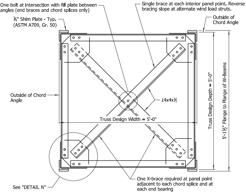
TRUSS SECTION Scale: 1" = 1'-0"
