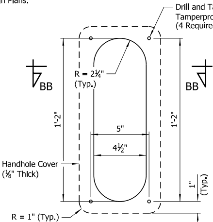
HANDHOLE DETAIL ② Scale: 3" = 1'-0"
