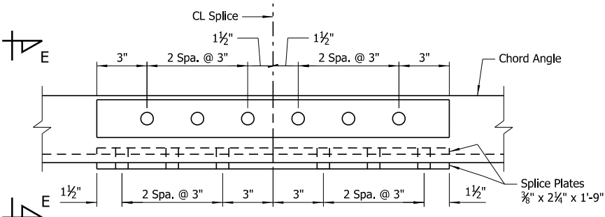
CHORD SPLICE Scale: 3" = 1'-0"
