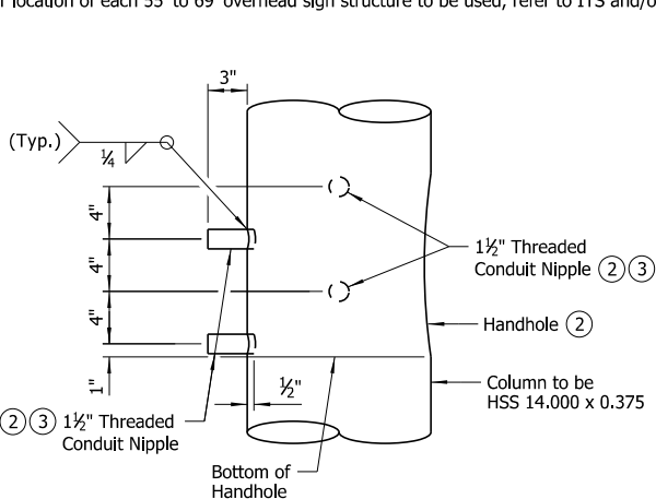
DETAIL P Scale: 1\frac{1}{2} " = 1'-0"
