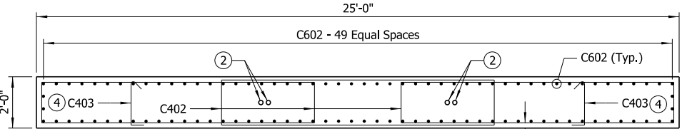
SECTION F-F Scale: \frac{3}{8} " = 1'-0"
