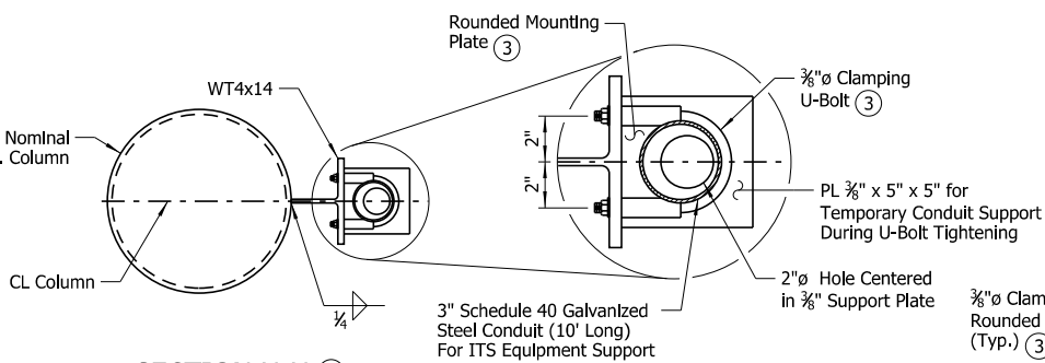
SECTION U-U ④ Scale: 1 1/2" = 1'-0"
