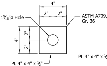
ELEVATION - COLUMN BASE Scale: 1" = 1'-0"
