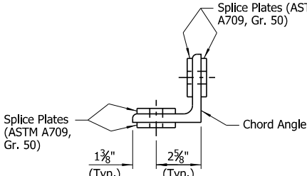
VIEW E-E Scale: 3" = 1'-0"
