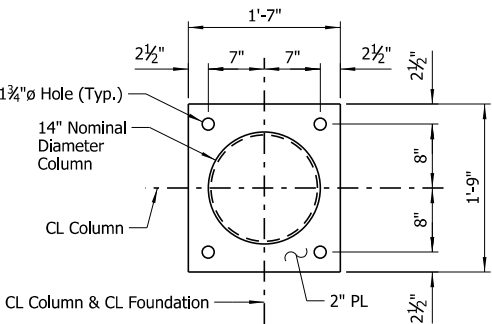
PLAN - COLUMN BASE Scale: 1" = 1'-0"
